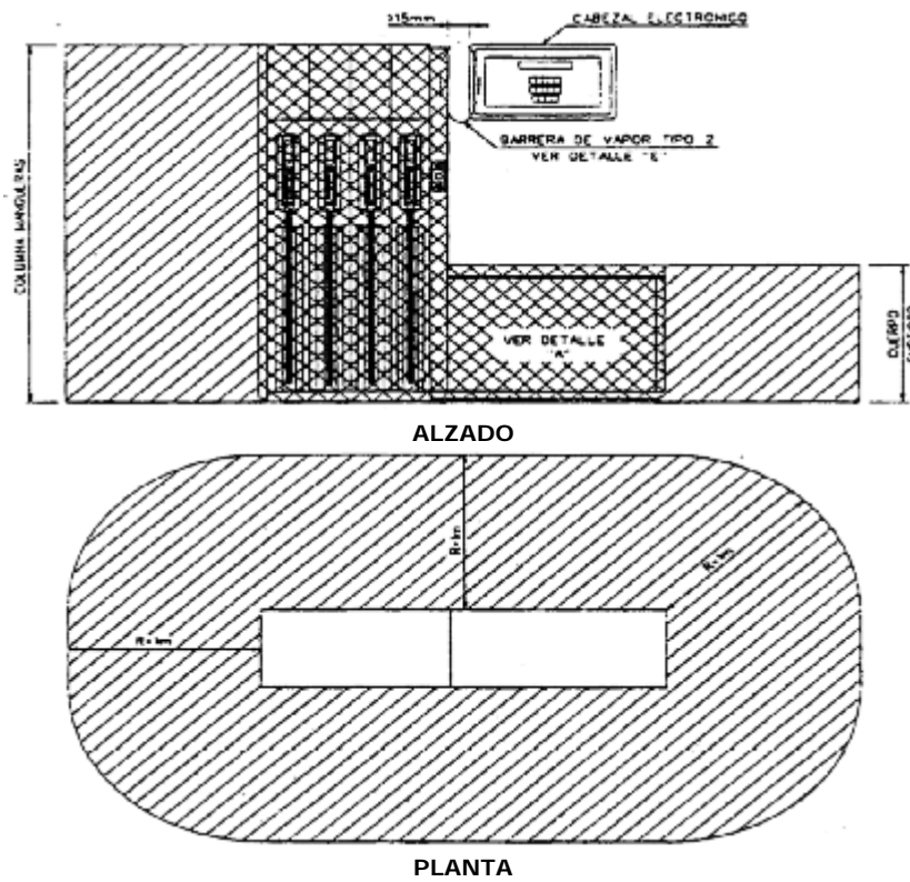
FIG. 4 SURTIDOR CON EL CABEZAL ELECTRONICO ELEVADO Y SEPARADO DE LA COLUMNA DE MANGUERAS A UNA DISTANCIA NO INFERIOR A 15 mm (BARRERA DE VAPOR TIPO 2)
