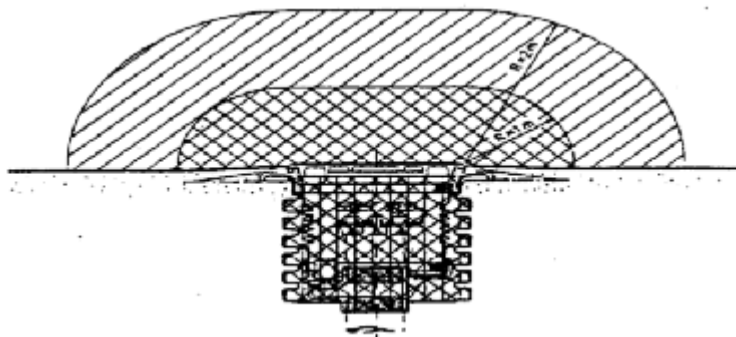
FIG. 5 DETALLES TÍPICOS DE LA CLASIFICACIÓN EN ARQUETAS
