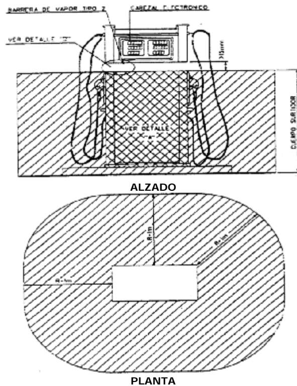
FIG. 3 SURTIDOR CON EL CABEZAL ELECTRONICO SEPARADO DE SU CUERPO UNA DISTANCIA NO INFERIOR A 15 mm (BARRERA DE VAPOR TIPO 2)
