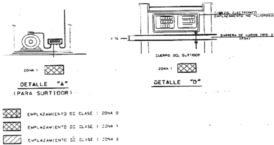
FIG. 4 SURTIDOR CON EL CABEZAL ELECTRONICO ELEVADO Y SEPARADO DE LA COLUMNA DE MANGUERAS A UNA DISTANCIA NO INFERIOR A 15 mm (BARRERA DE VAPOR TIPO 2)
