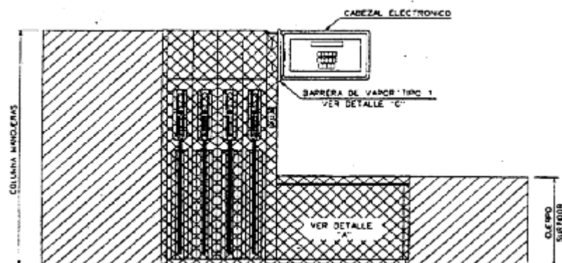
FIG. 2 SURTIDOR CON CABEZAL ELECTRÓNICO ELEVADO Y ADOSADO A LA COLUMNA DE MANGUERAS (BARRERA DE VAPOR TIPO 1)
